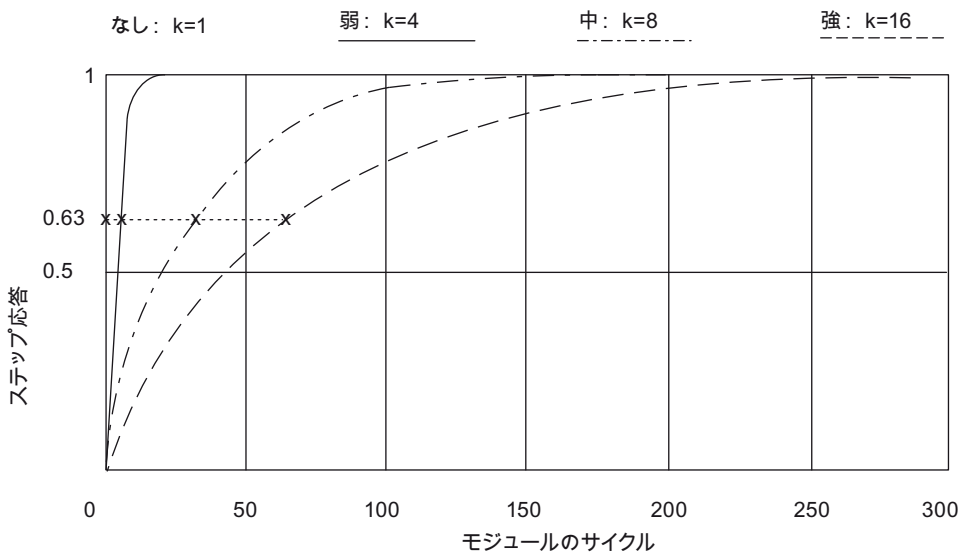
図 4-1 AI 4xI 2-/4-wire ST による平滑化
