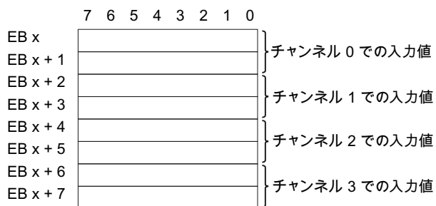
図 4-2 アナログ入力モジュール AI 4xI 2-/4-wire ST のアドレス空間
