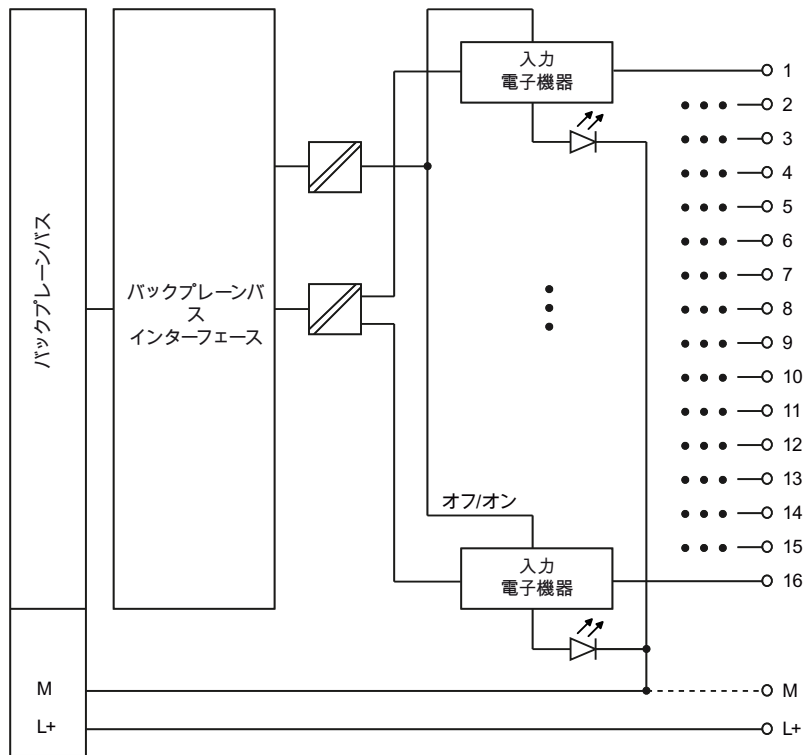
図 3-1 DI 16x24VDC ST の回路概略図
