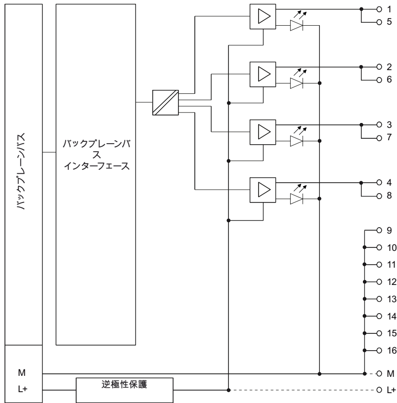
図 3-1 DQ 4x24VDC/2A ST の回路概略図
