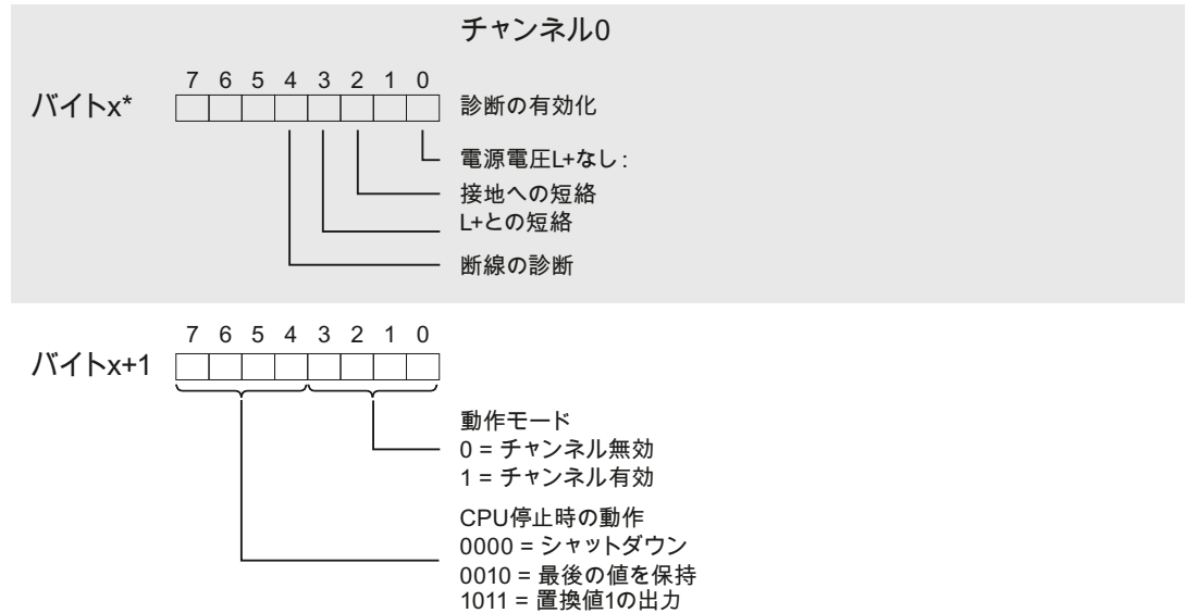
図 A-3 構造バイト x~x+1、チャンネル 0~3 用
