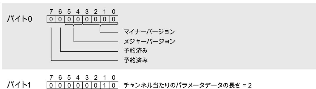
図 A-2 ヘッダー情報
