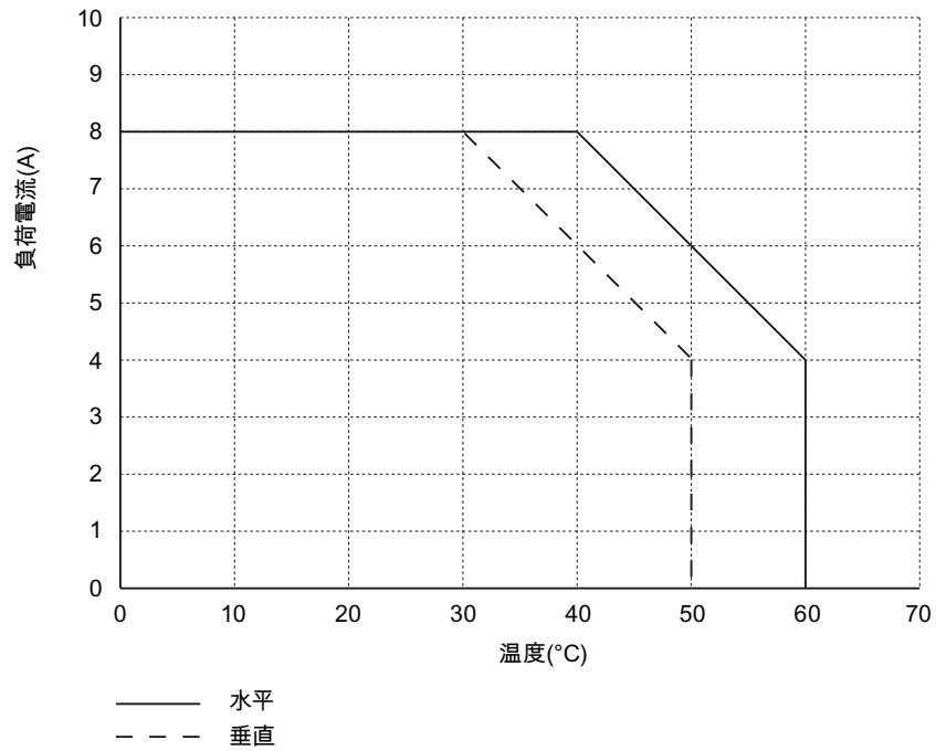
図 6-1 取り付け位置に対する負荷電流
